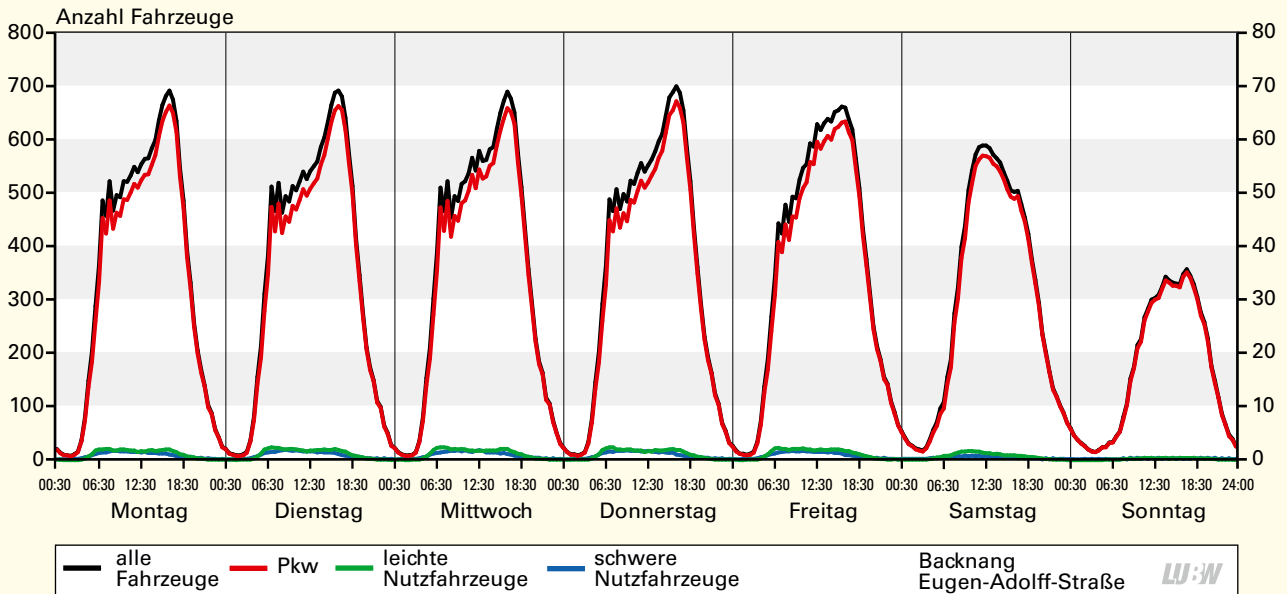
Mittlerer Wochengang der Verkehrsstärken der 3 Fahrzeugklassen an der Verkehrszählstelle Backnang Eugen-Adolff-Straße 2021; Basis: Halbstundenwerte
