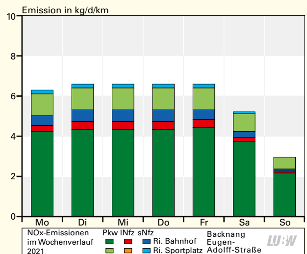
Mittlerer Wochengang der NO x -Emissionen nach Fahrzeugklassen und Fahrtrichtungen an der Verkehrszählstelle Backnang Eugen-Adolff-Straße 2021
