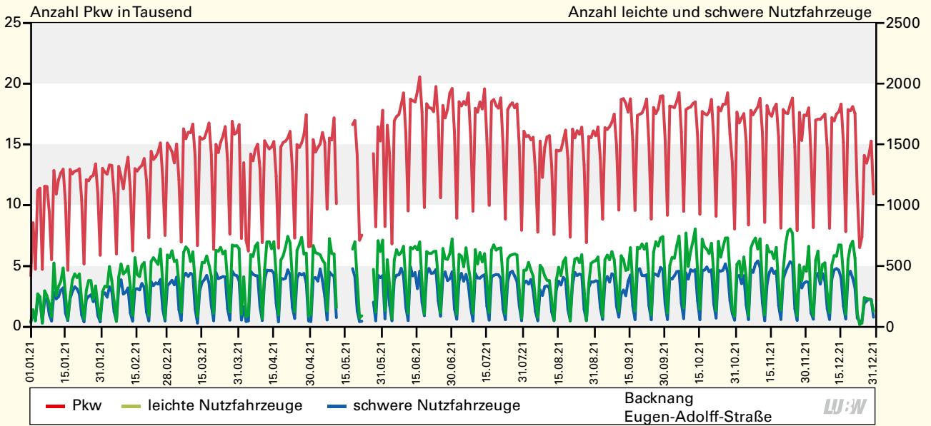
Verlauf der täglichen Verkehrsstärken der 3 Fahrzeugklassen am Standort Backnang Eugen-Adolff-Straße 2021
