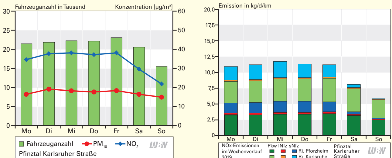
Mittlerer Wochengang der Gesamtverkehrsstärke, Stickstoffdioxid- und Partikel PM 10 -Konzentration an der Verkehrszählstelle Pfinztal Karlsruhe Straße 2019; Basis: Tagesmittelwerte
