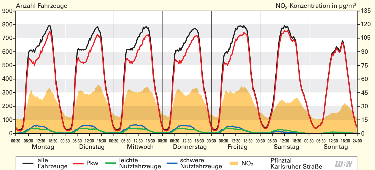
Mittlerer Wochengang der Verkehrsstärken der 3 Fahrzeugklassen sowie der Stickstoffdioxidkonzentration an der Verkehrszählstelle Pfinztal Karlsruhe Straße 2019; Basis: Halbstundenwerte
