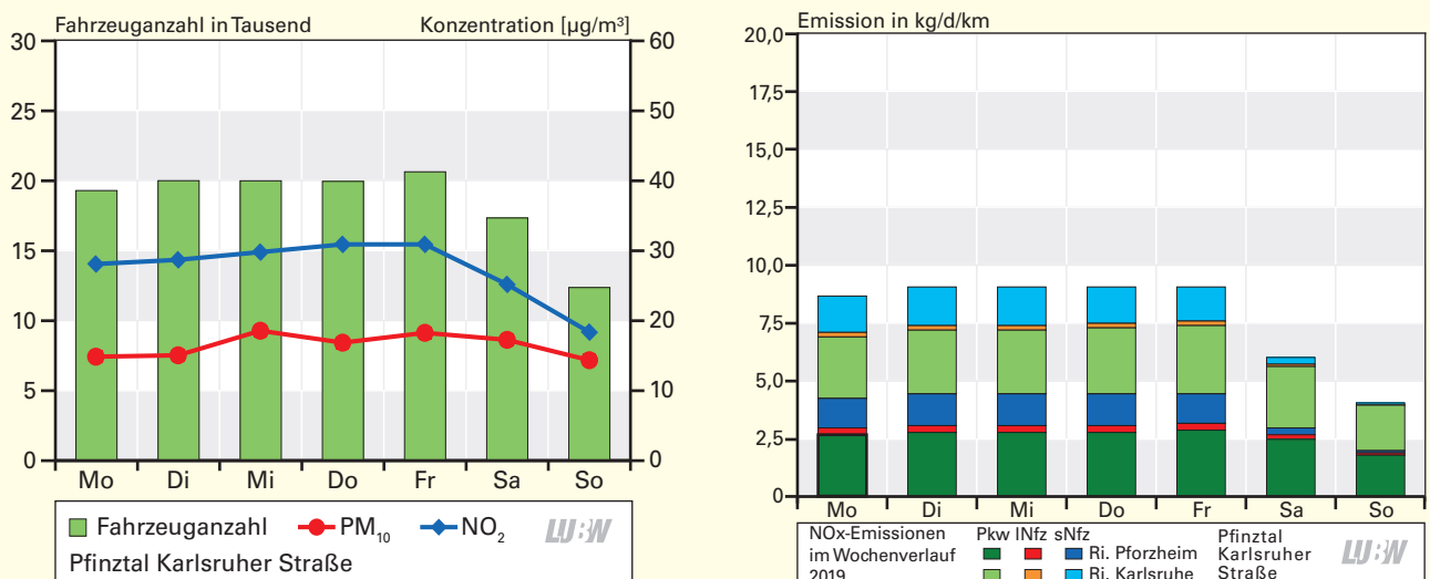
Mittlerer Wochengang der Gesamtverkehrsstärke, Stickstoffdioxid- und Partikel PM 10 -Konzentration an der Verkehrszählstelle Pfinztal Karlsruher Straße 2020; Basis: Tagesmittelwerte
