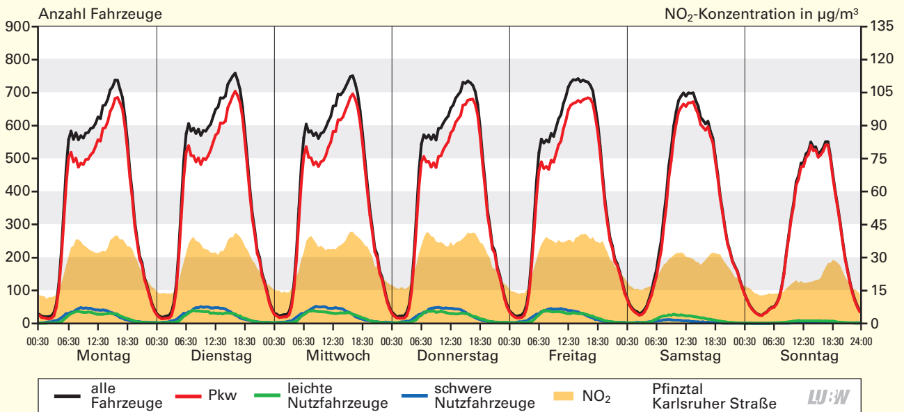
Mittlerer Wochengang der Verkehrsstärken der 3 Fahrzeugklassen sowie der Stickstoffdioxidkonzentration an der Verkehrszählstelle Pfinztal Karlsruher Straße 2020; Basis: Halbstundenwerte
