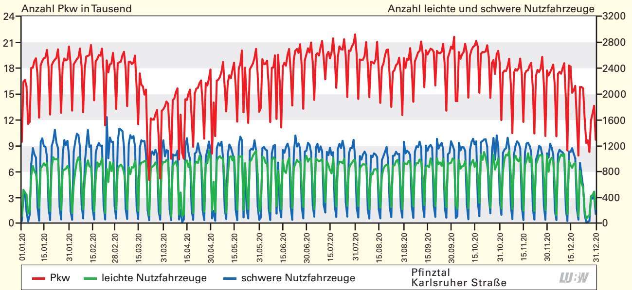
Verlauf der täglichen Verkehrsstärken der 3 Fahrzeugklassen am Standort Pfinztal Karlsruher Straße 2020
