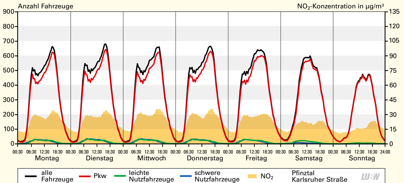
Mittlerer Wochengang der Verkehrsstärken der 3 Fahrzeugklassen an der Verkehrszählstelle Pfinztal Karlsruher Straße 2021; Basis: Halbstundenwerte
