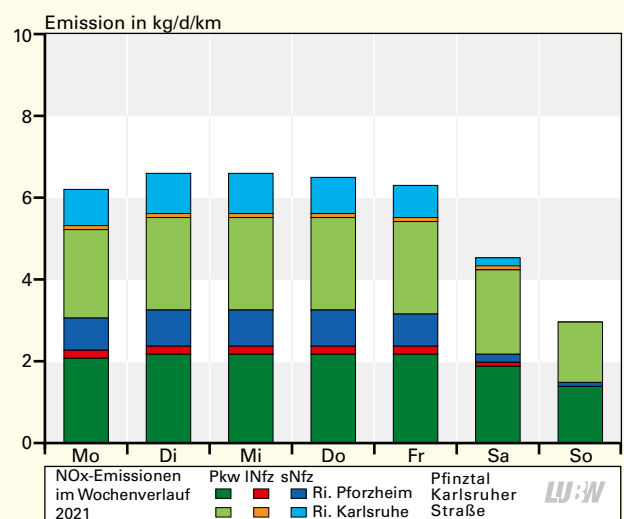
Mittlerer Wochengang der NO x -Emissionen nach Fahrzeugklassen und Fahrtrichtungen an der Verkehrszählstelle Pfinztal Karlsruher Straße 2021
