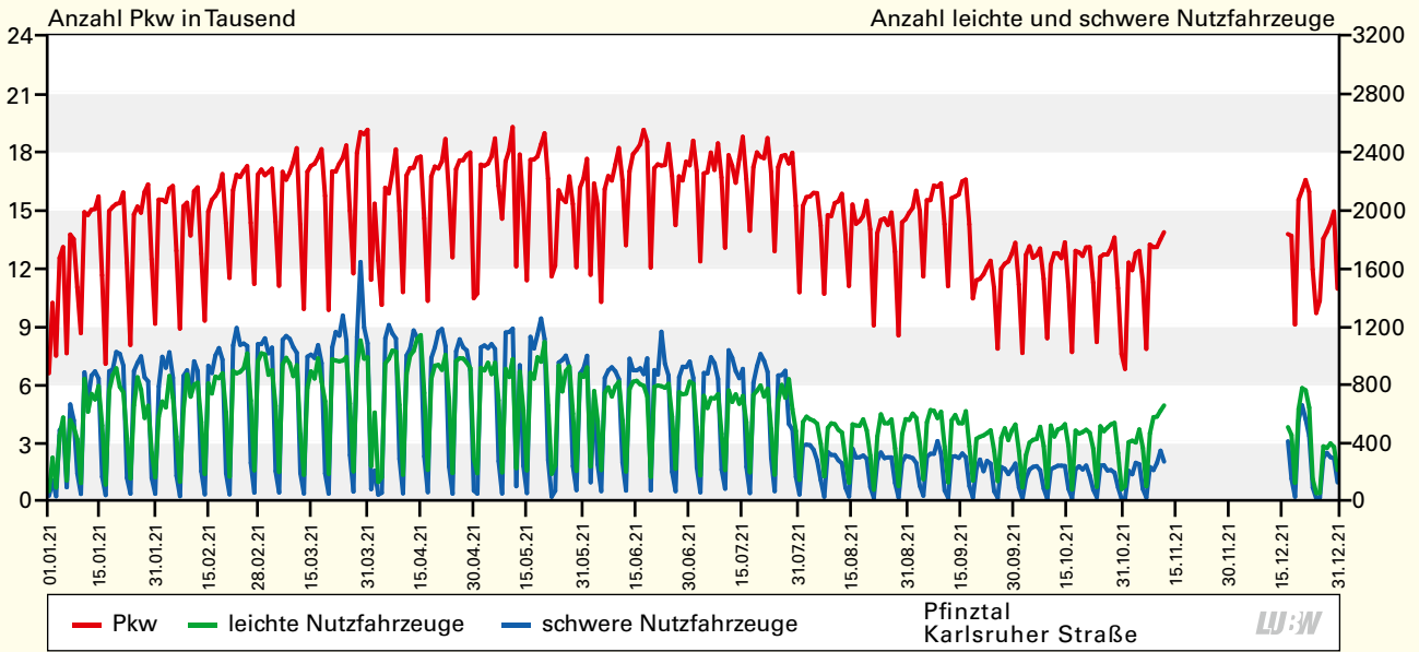
Verlauf der täglichen Verkehrsstärken der 3 Fahrzeugklassen am Standort Pfinztal Karlsruher Straße 2021
