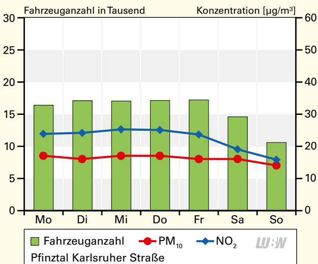
Mittlerer Wochengang der Gesamtverkehrsstärke, Stickstoffdioxid- und Feinstaub PM 10 -Konzentration an der Verkehrszählstelle Pfinztal Karlsruher Straße 2021; Basis: Tagesmittelwerte
