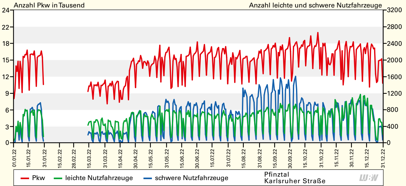
Verlauf der täglichen Verkehrsstärken der 3 Fahrzeugklassen am Standort Pfinztal Karlsruher Straße 2022
