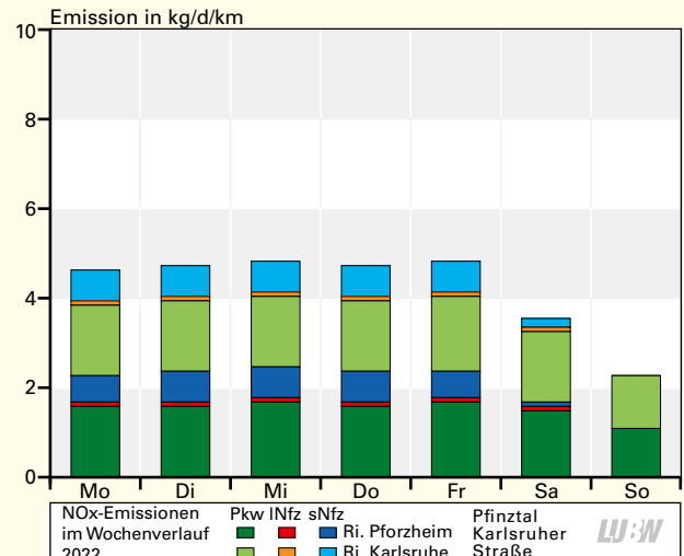
Mittlerer Wochengang der NO x -Emissionen nach Fahrzeugklassen und Fahrrichtungen an der Verkehrszählstelle Pfinztal Karlsruher Straße 2022
