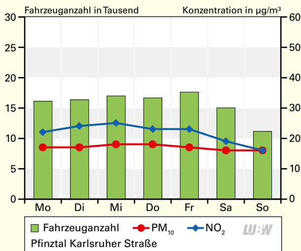
Mittlerer Wochengang der Gesamtverkehrsstärke, Stickstoffdioxid- und Feinstaub PM 10 -Konzentration an der Verkehrszählstelle Pfinztal Karlsruher Straße 2022; Basis: Tagesmittelwerte
