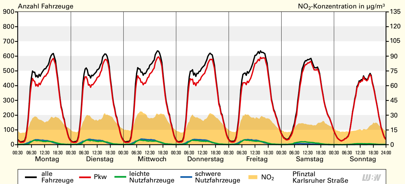
Mittlerer Wochengang der Verkehrsstärken der 3 Fahrzeugklassen sowie der Stickstoffdioxid-Konzentration an der Verkehrszählstelle Pfinztal Karlsruher Straße 2022; Basis: Halbstundenwerte
