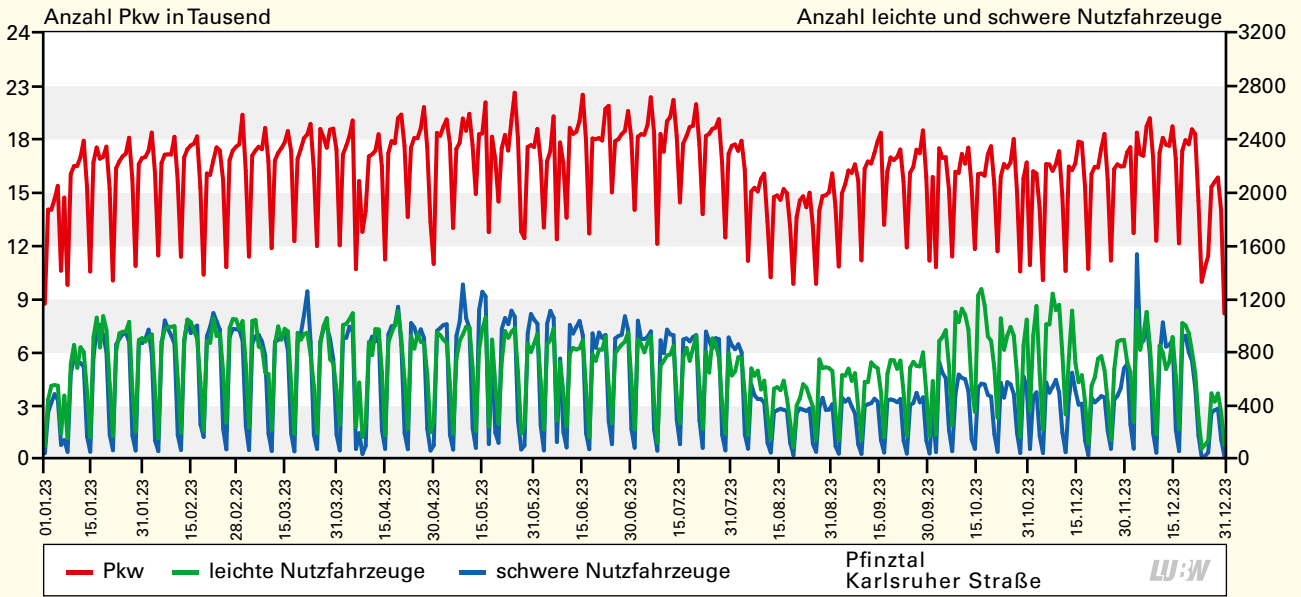
Verlauf der täglichen Verkehrsstärken der 3 Fahrzeugklassen am Standort Pfinztal Karlsruhe Straße 2023
