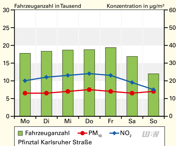
Mittlerer Wochengang der Gesamtverkehrsstärke, Stickstoffdioxid- und Feinstaub PM 10 -Konzentration an der Verkehrszählstelle Pfinztal Karlsruhe Straße 2023; Basis: Tagesmittelwerte
