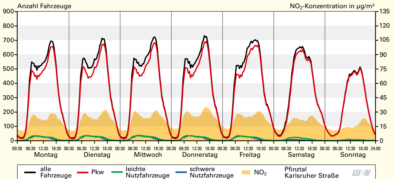
Mittlerer Wochengang der Verkehrsstärken der 3 Fahrzeugklassen sowie der Stickstoffdioxid-Konzentration an der Verkehrszählstelle Pfinztal Karlsruhe Straße 2023; Basis: Halbstundenwerte
