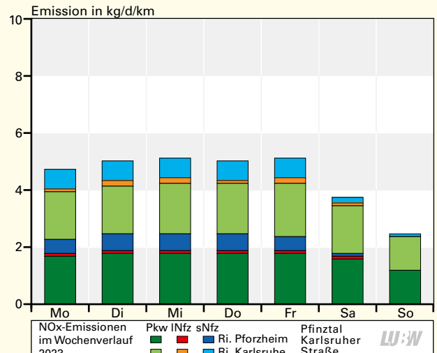
Mittlerer Wochengang der NO x -Emissionen nach Fahrzeugklassen und Fahrtrichtungen an der Verkehrszählstelle Pfinztal Karlsruhe Straße 2023
