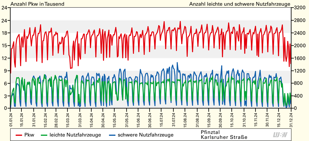
Verlauf der täglichen Verkehrsstärken der 3 Fahrzeugklassen am Standort Pfinztal Karlsruhe Straße 2024
