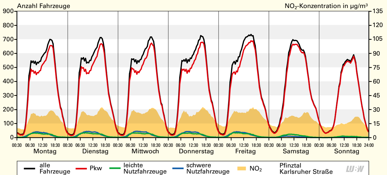
Mittlerer Wochengang der Verkehrsstärken der 3 Fahrzeugklassen sowie der Stickstoffdioxid-Konzentration an der Verkehrszählstelle Pfinztal Karlsruhe Straße 2024; Basis: Halbstundenwerte
