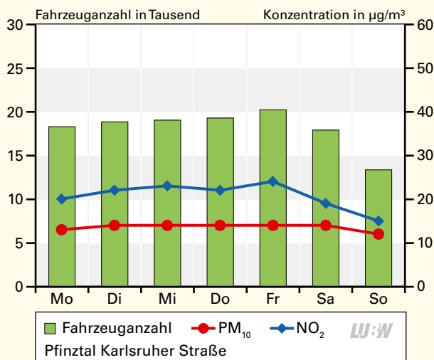
Mittlerer Wochengang der Gesamtverkehrsstärke, Stickstoffdioxid- und Feinstaub PM 10 -Konzentration an der Verkehrszählstelle Pfinztal Karlsruhe Straße 2024; Basis: Tagesmittelwerte
