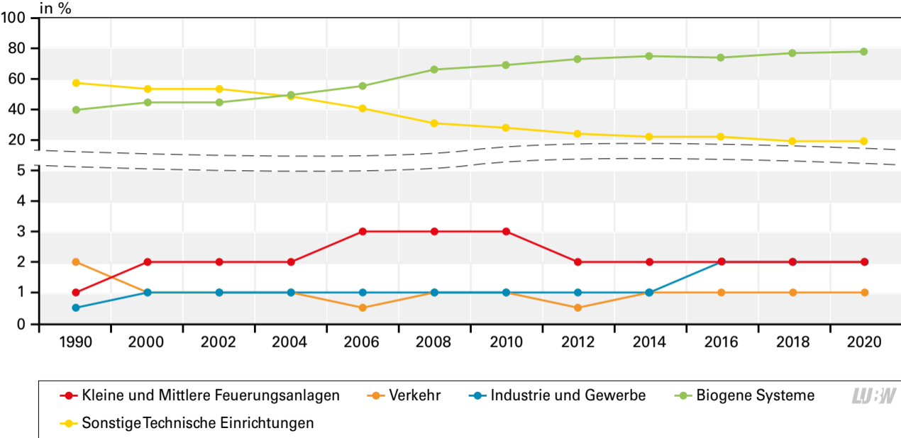
Entwicklung der jährlichen CH 4 -Emissionen in Baden-Württemberg von 1990 bis 2020
