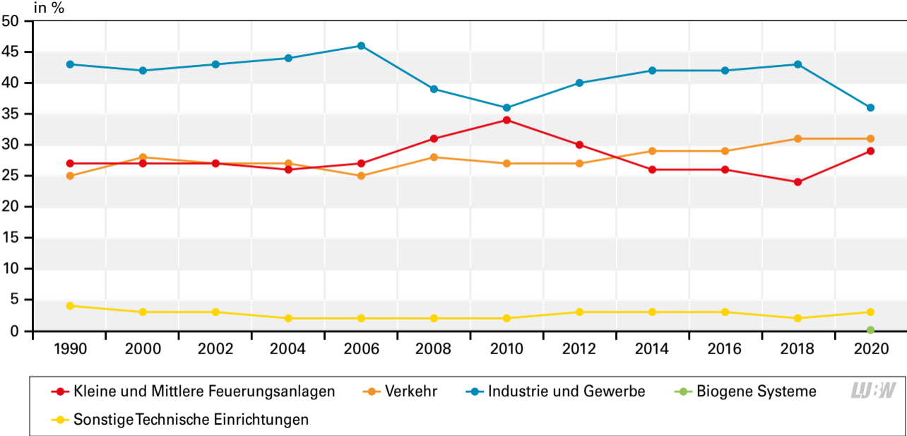
Entwicklung der jährlichen CO 2 -Emissionen in Baden-Württemberg von 1990 bis 2020
