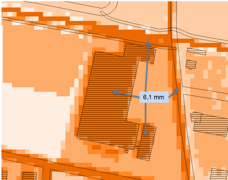
Abbildung 2: Teilausschnitt aus Abbildung 1. Zu erkennen sind die Übergangsbereiche an den Gebäuden und Straßen, die die Mittelwerte aus den vollversiegelten und nur teilweise oder gar nicht versiegelten Nachbarflächen abbilden. Zur Übertragung auf neu hinzugekommene Gebäude- und Straßenflächen sollten die Werte aus dem Zentrum der schon vorhandenen Geometrien verwendet werden, hier 6,1 mm.
