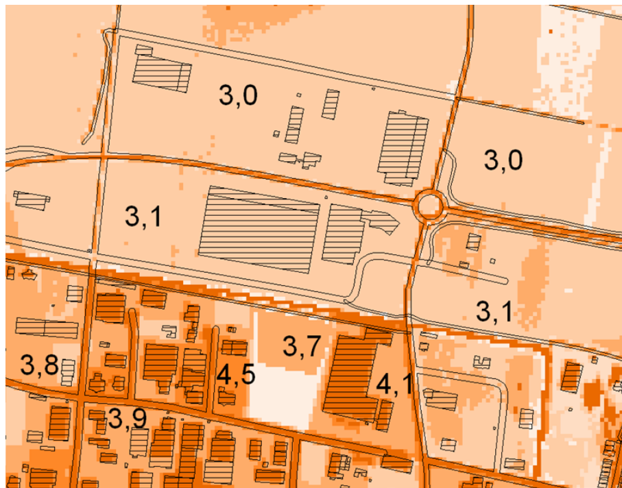
Abbildung 3: OAK-Werte [mm/5 min] auf den Grundstücken um die alte Bebauung und auf den Flächen, auf denen neue Gebäude errichtet wurden.
